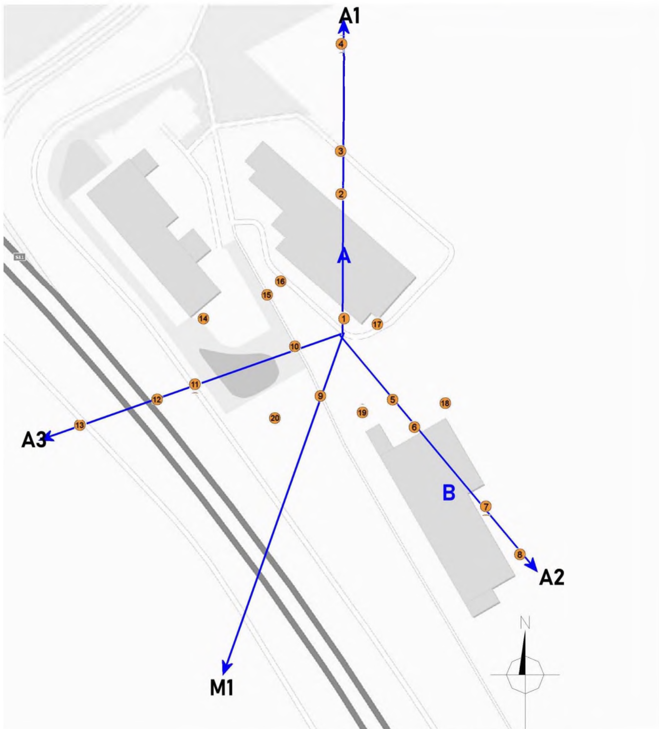
Azymuty anten Orange Polska S.A.
