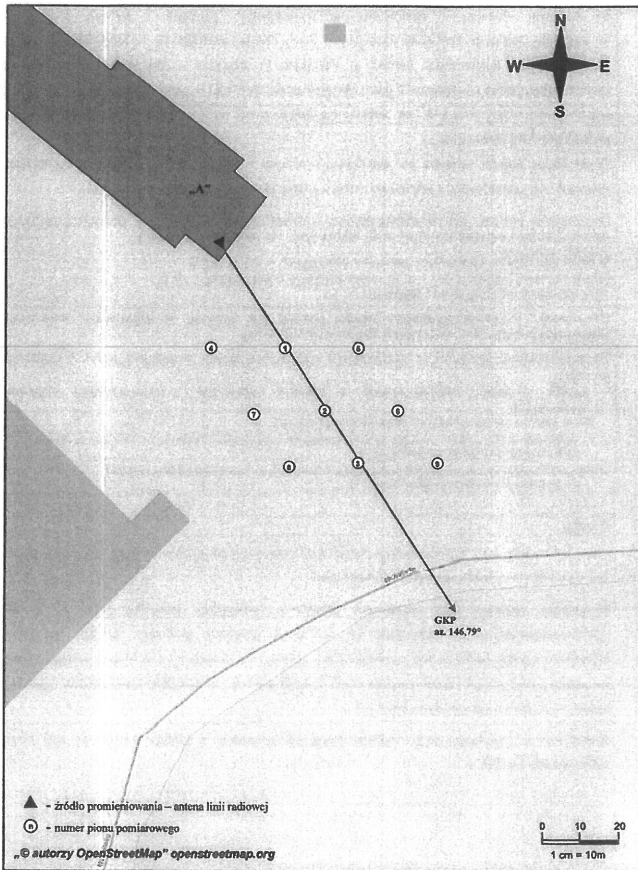
Rys. 1. Usytuowanie punktów i pionów pomiarowych w otoczeniu instalacji radiokomunikacyjnej Stacja Netia KORNB111-KORN00050ANT001 Żemiki, ul. Fabryczna 11
