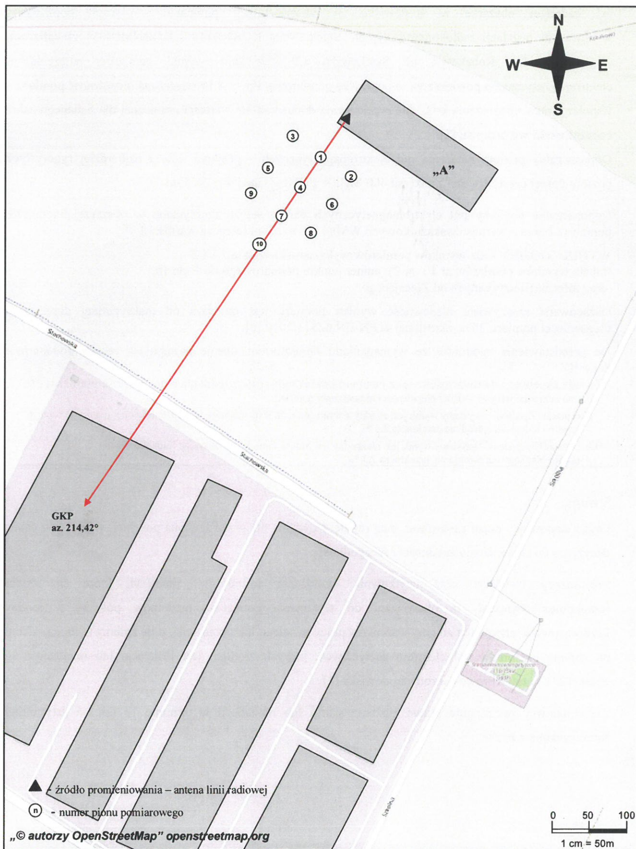
Rys. 1. Usytuowanie punktów i pionów pomiarowych w otoczeniu instalacji radiokomunikacyjnej Stacja Netia KORNB115-KORN00051 Robakowo, ul. Stachowska 17F
