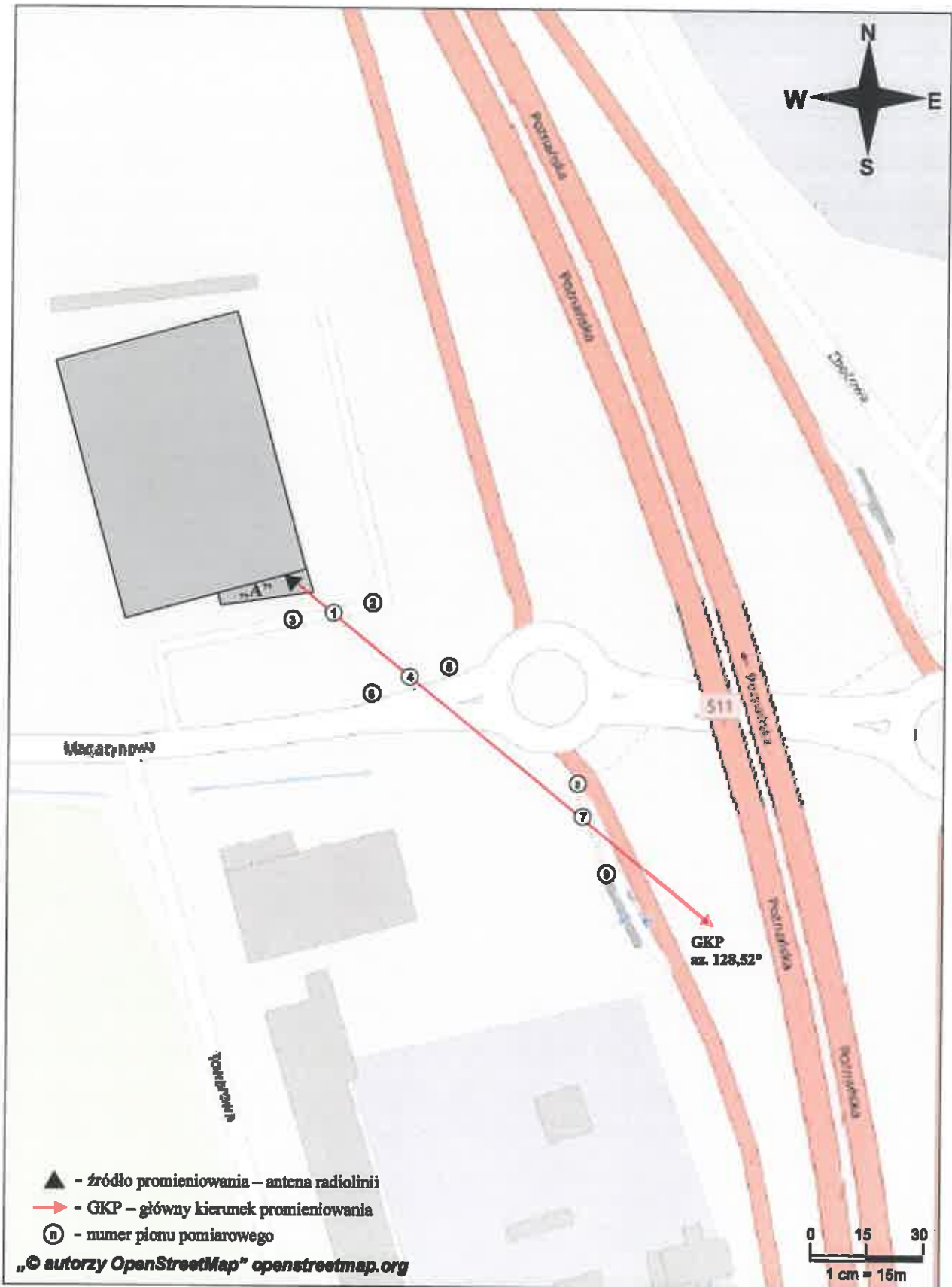
Rys. 1. Usytuowanie punktów i pionów pomiarowych w otoczeniu instalacji radiokomunikacyjnej Stacja Netia KORNB026-KORNM00014 Gądky, ul. Magazynowa 19
