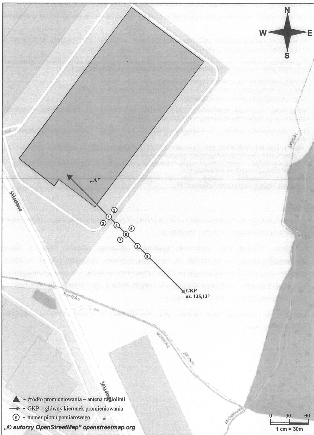
Rys. 1. Usytuowanie punktów i pionów pomiarowych w otoczeniu instalacji radiokomunikacyjnej Stacja Netia KORNB122-KORNM00053 Żerniki, ul. Składowa 4c
