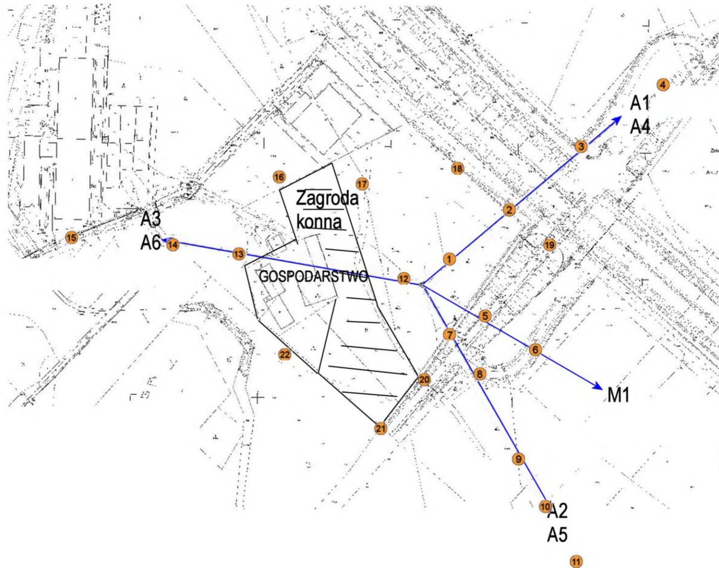
Azymuty anten T-Mobile
