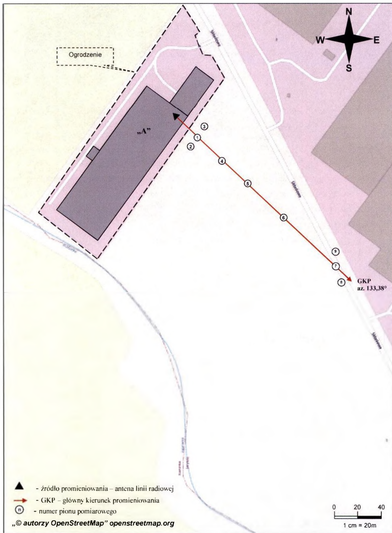
Rys. 1. Usytuowanie punktów i pionów pomiarowych w otoczeniu instalacji radiokomunikacyjnej Stacja Netia KORNB131-KORNM00055 Żerniki, ul. Składowa 7
