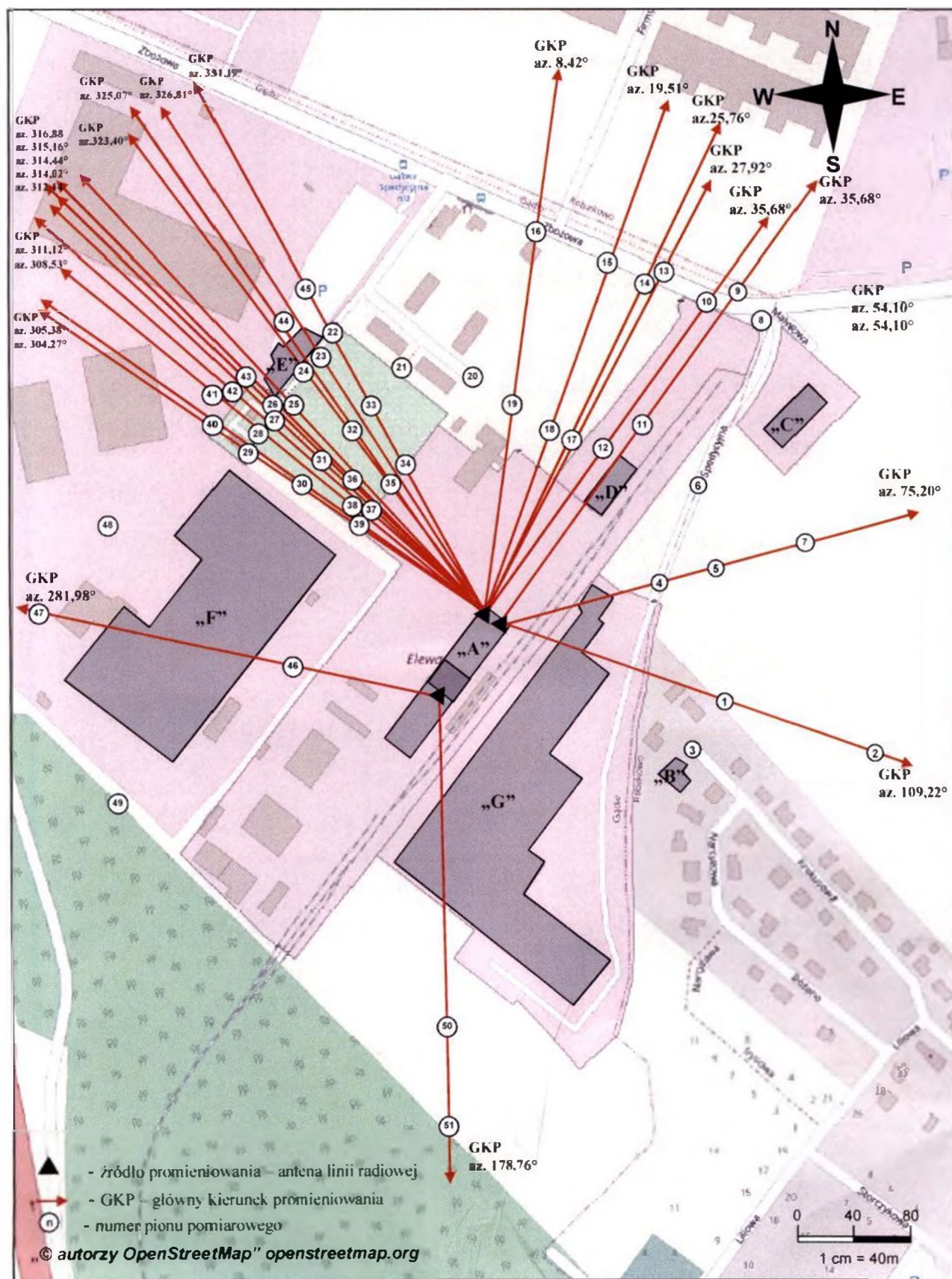
Rys. 1. Usytuowanie punktów i pionów pomiarowych w otoczeniu instalacji radiokomunikacyjnej Stacja Netia KORNT001-KORNM00001 Gądk, ul. Zbożowa 1
