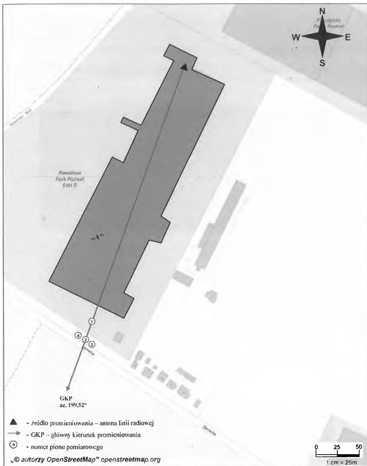
Rys. 1. Usytuowanie punktów i pionów pomiarowych w otoczeniu instalacji radiokomunikacyjnej Stacja Netia KORNB150-KORNM00063 Robakowo, ul. Żernicka 12
