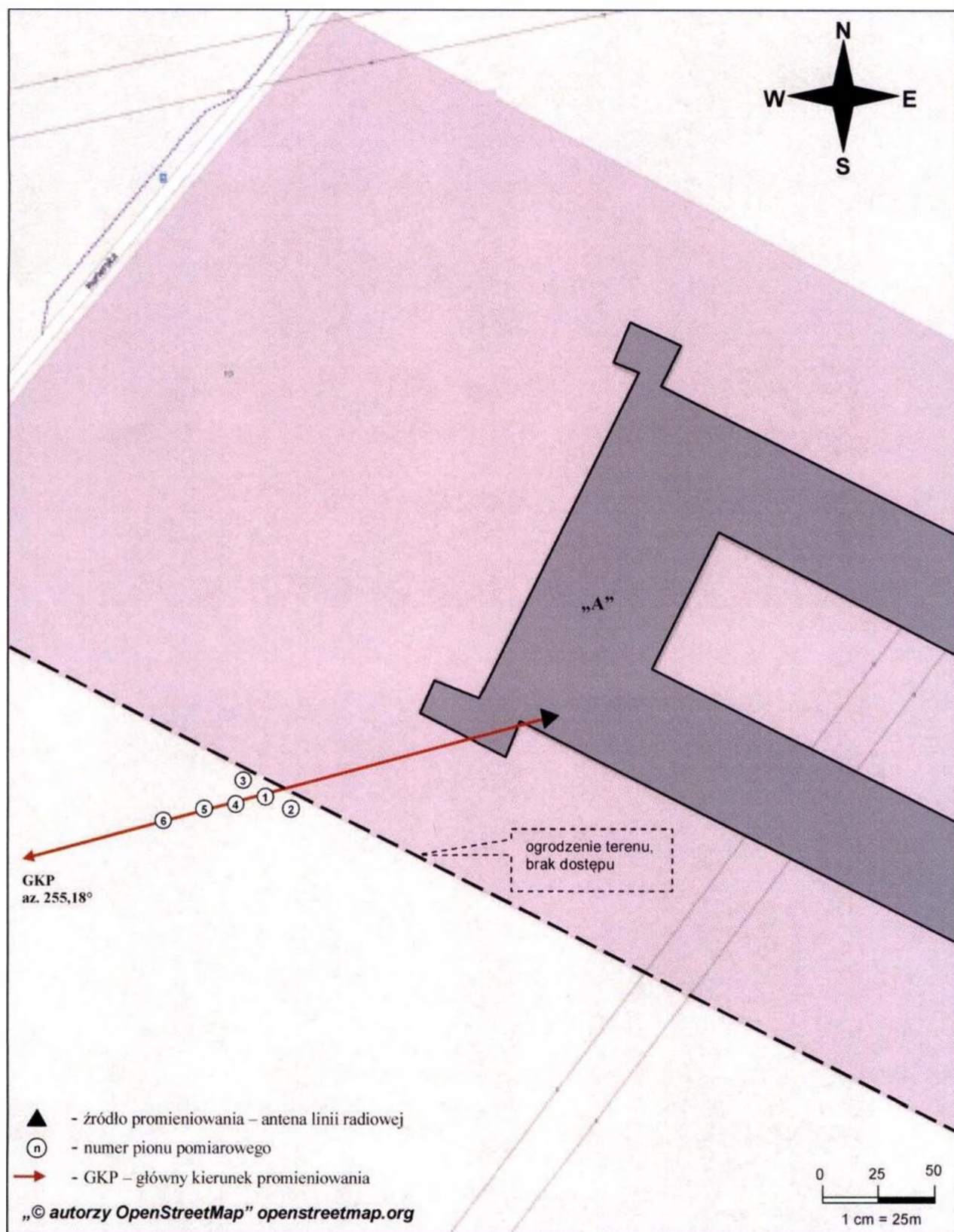
Rys. 1. Usytuowanie punktów i pionów pomiarowych w otoczeniu instalacji radiokomunikacyjnej Stacja Netia KORNB141-KORNM00060 Robakowo, ul. Kurierska 10
