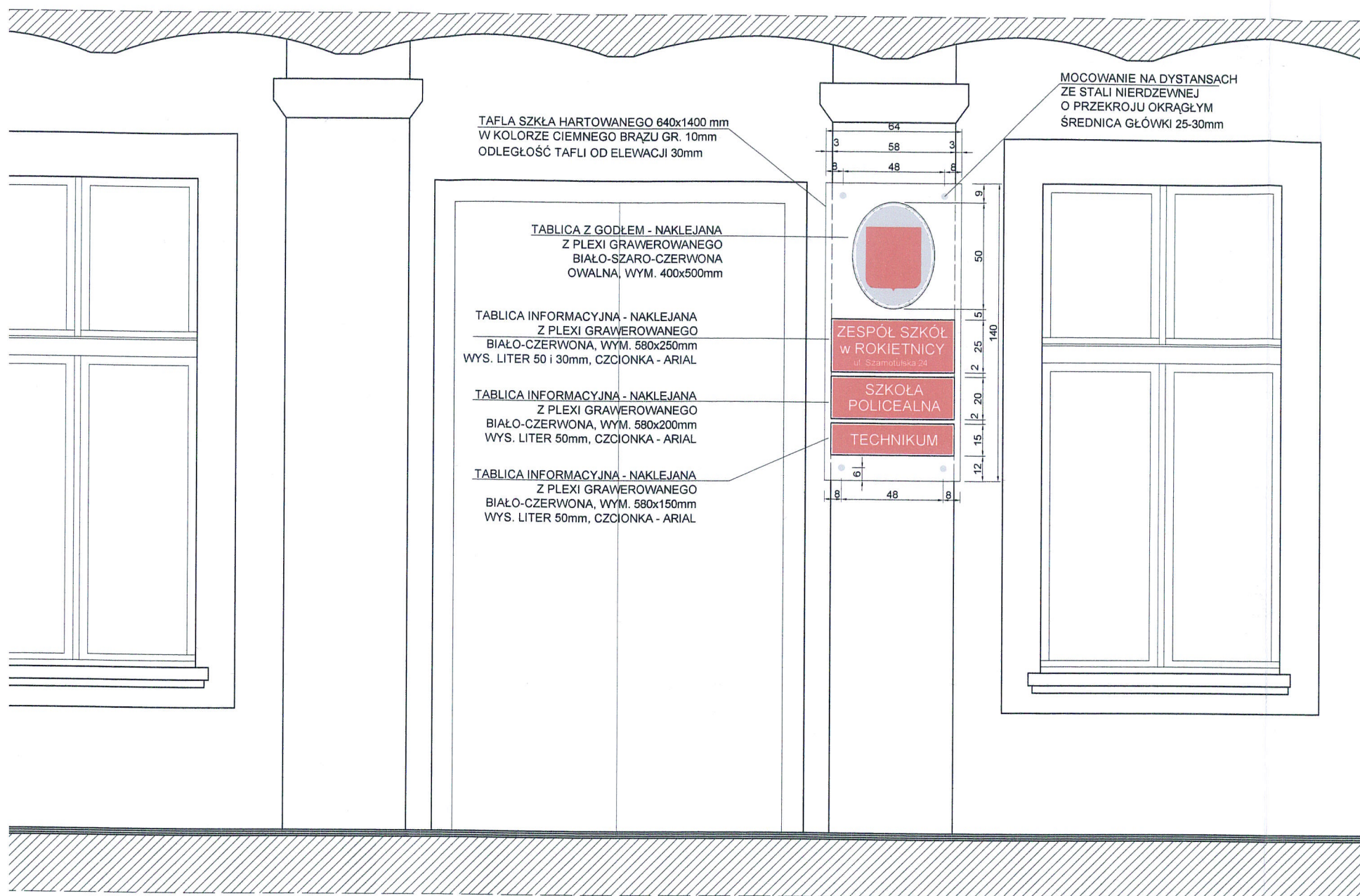
ŚCIANA FRONTOWA
