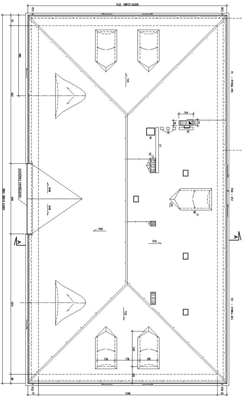
RZUT DACHU 1:50
