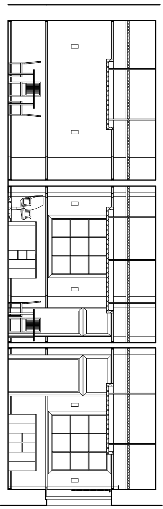
PRZEKROJ 5-5
