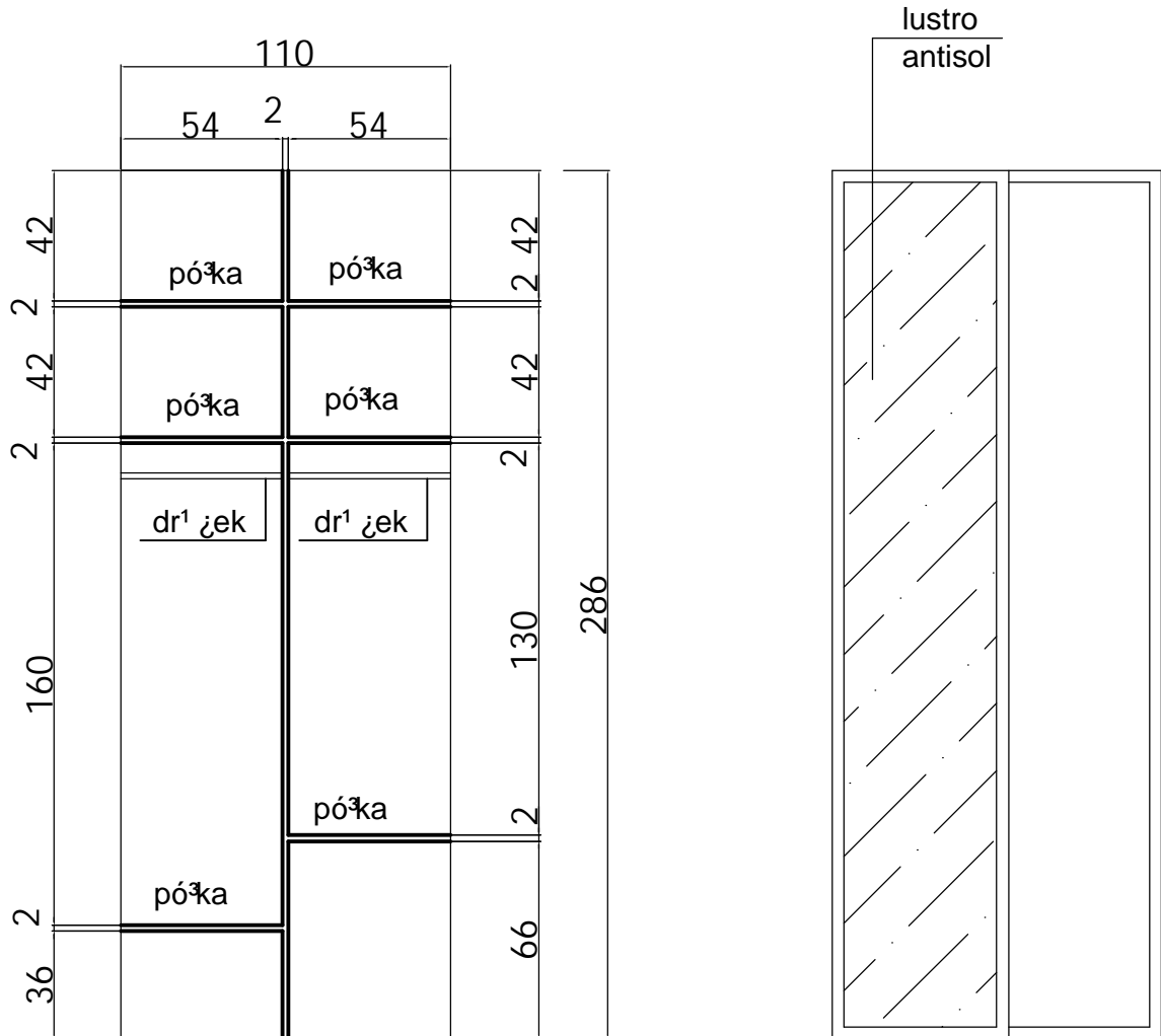
PRZEKRÓJ
