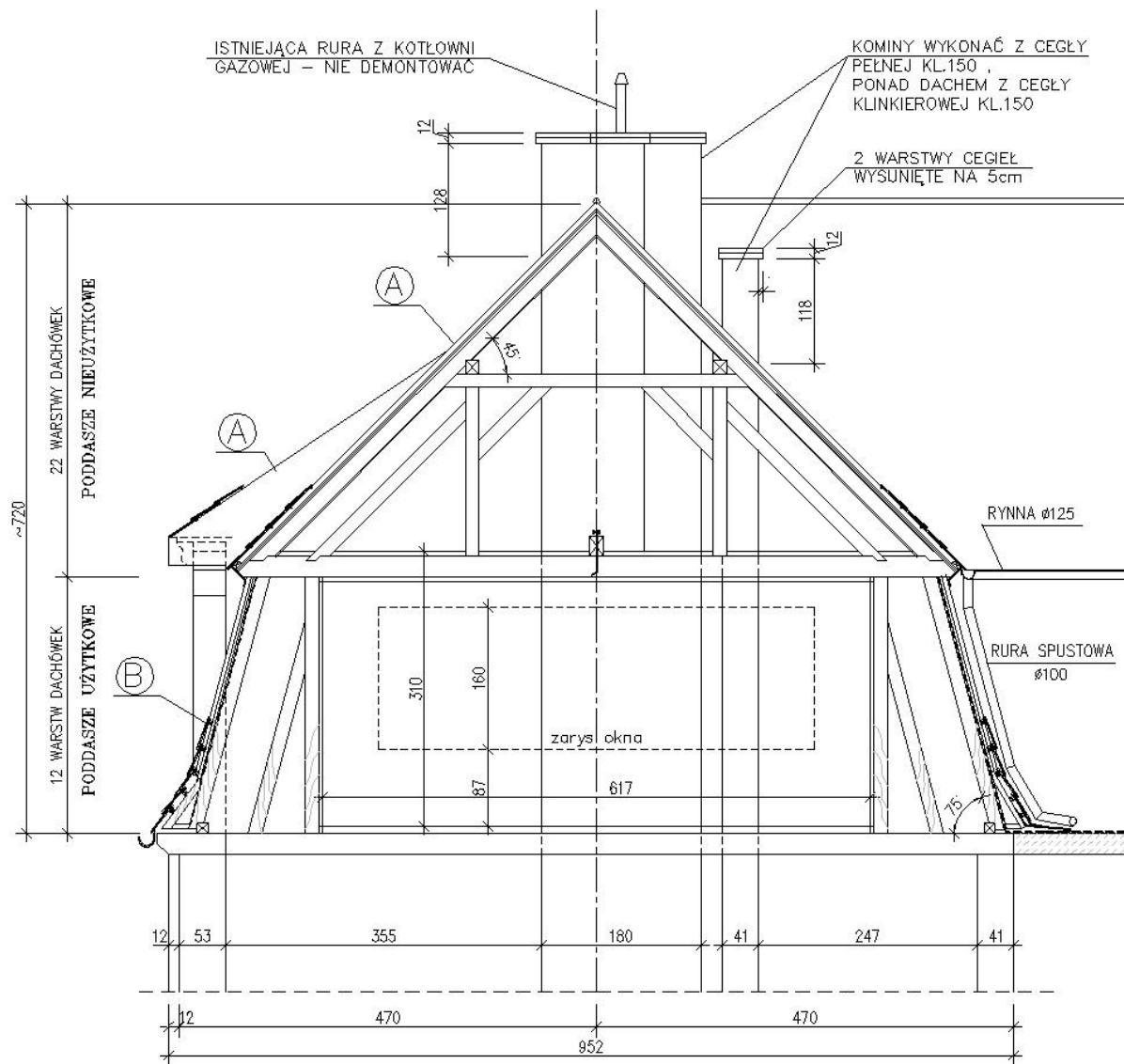
PRZEKRÓJ A-A
