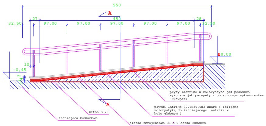
PRZEKRÓJ B-B
