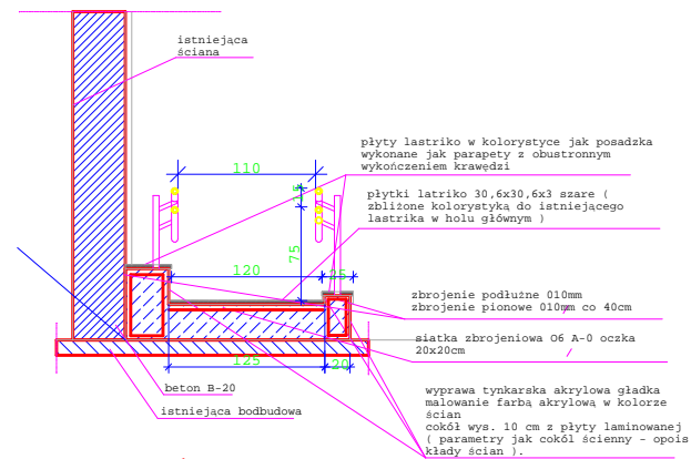
PRZEKRÓJ A-A
